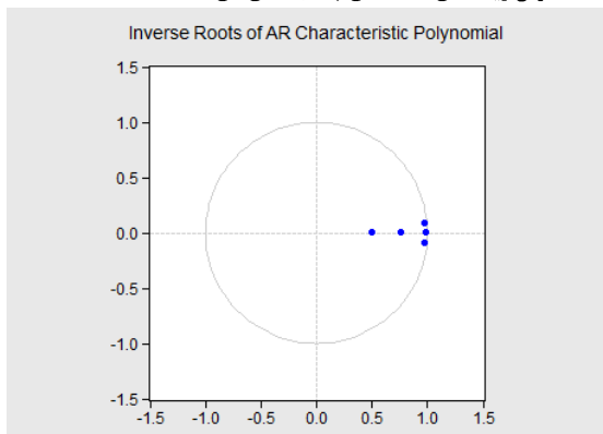
نمودار (۱): معکوس ریشه‌های مشخصی چندجمله‌ای‌های AR
