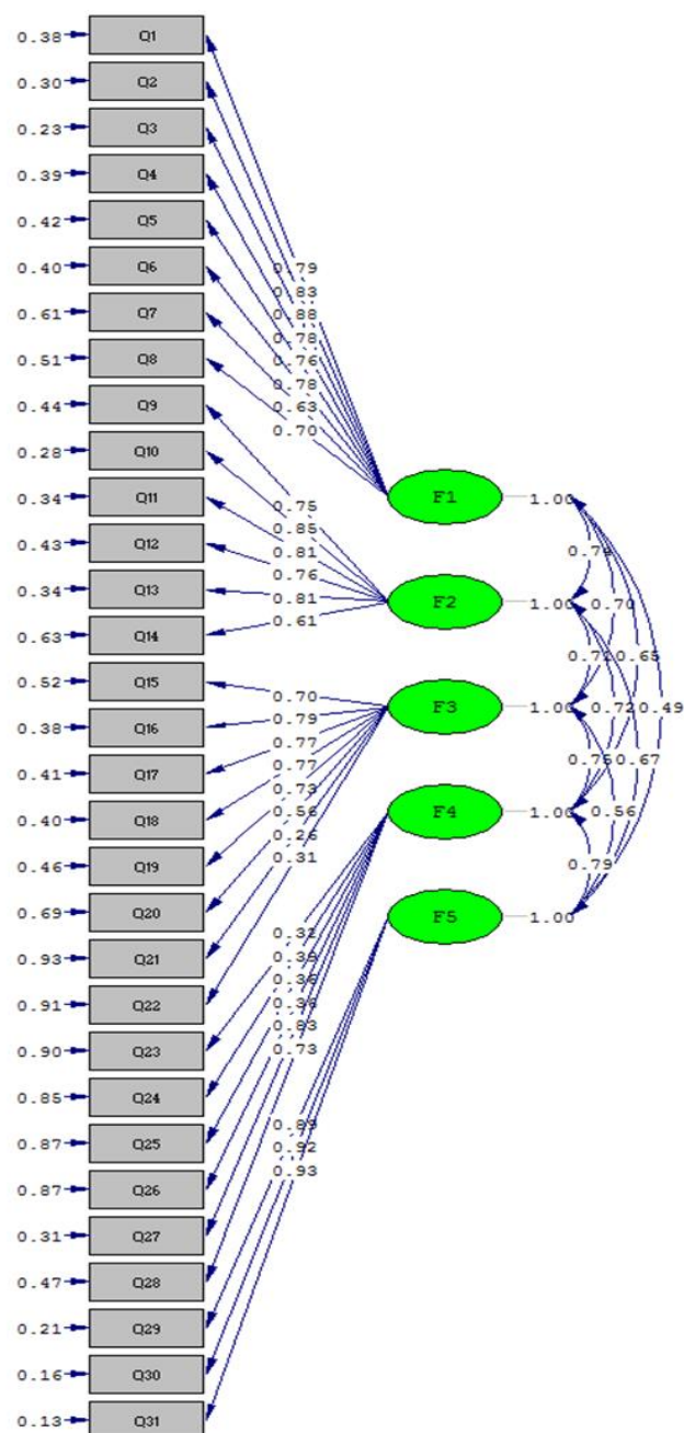
شکل ۱: نمودار تحلیلی عاملی تأییدی
