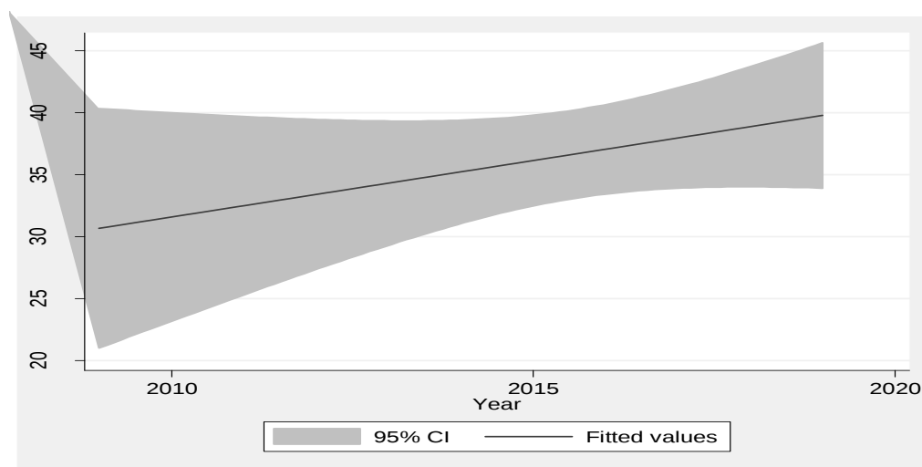
شکل ۳ الف: متارگرسیون مطالعات بر حسب سال
