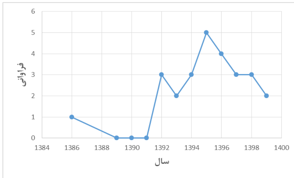
نمودار ۲. فراوانی انتشار مقالات بر حسب زمان
