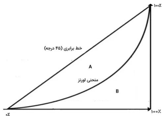
شکل ۱: منحنی لورنز
